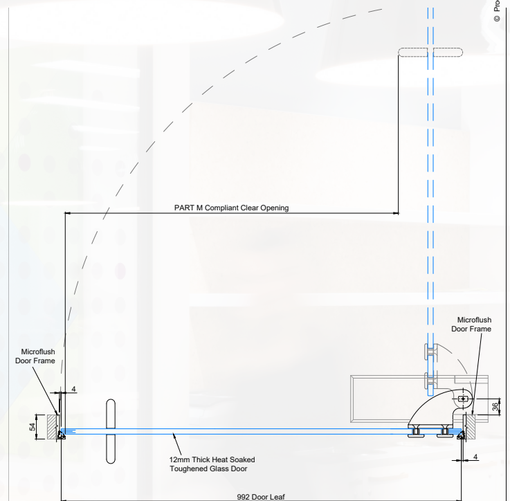
AXILE PULSE INLINE PIVOTING DOOR
